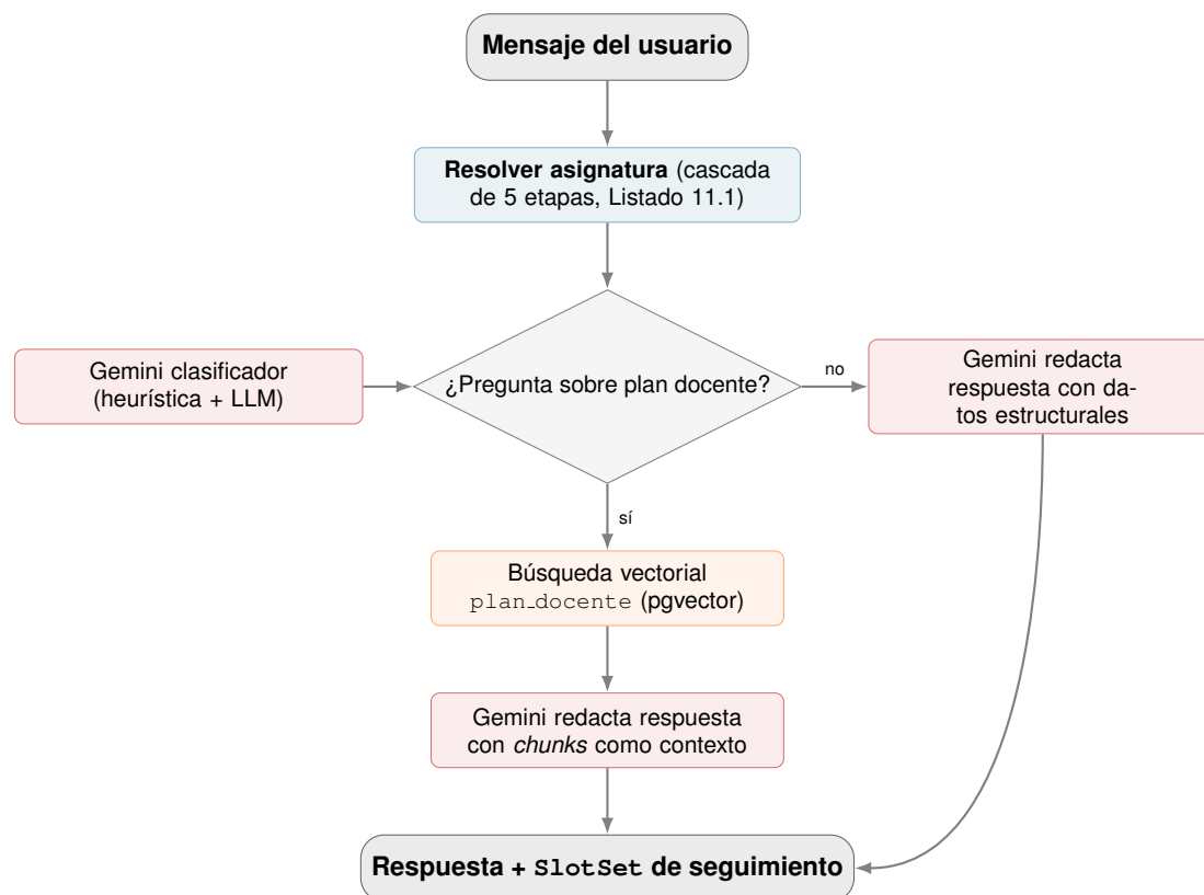
Figura 11.1: Pipeline de ActionConsultaEspecificas . La caja Resolver asignatura encapsula la cascada de cinco estrategias detallada en el Listado 11.1.
